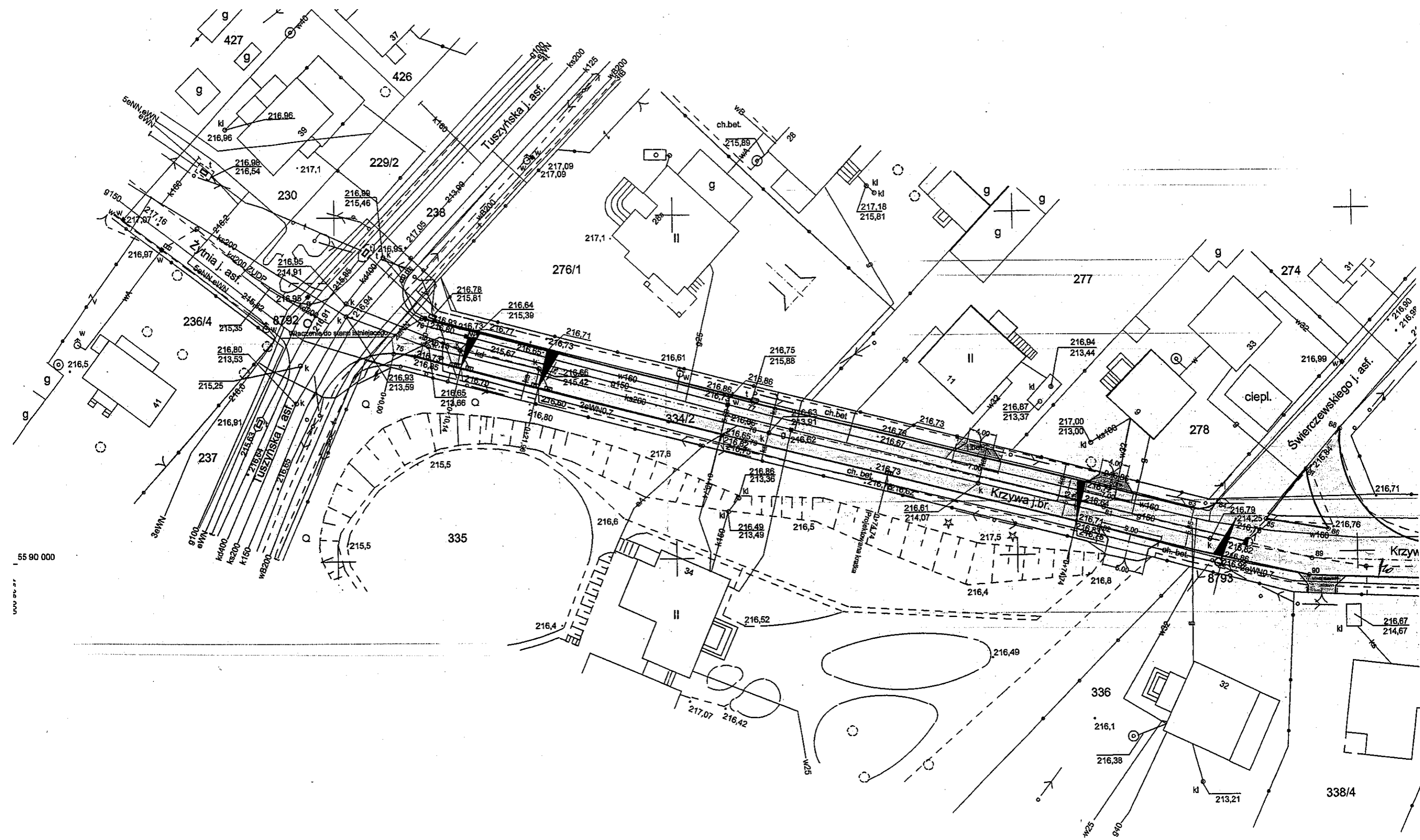
Plan sytuacyjno - wysokościowy
